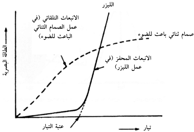
الشكل 4-8 مقارنة بين الخصائص البصرية للصبامات الثنائية الباعثة للضوء والليزر
